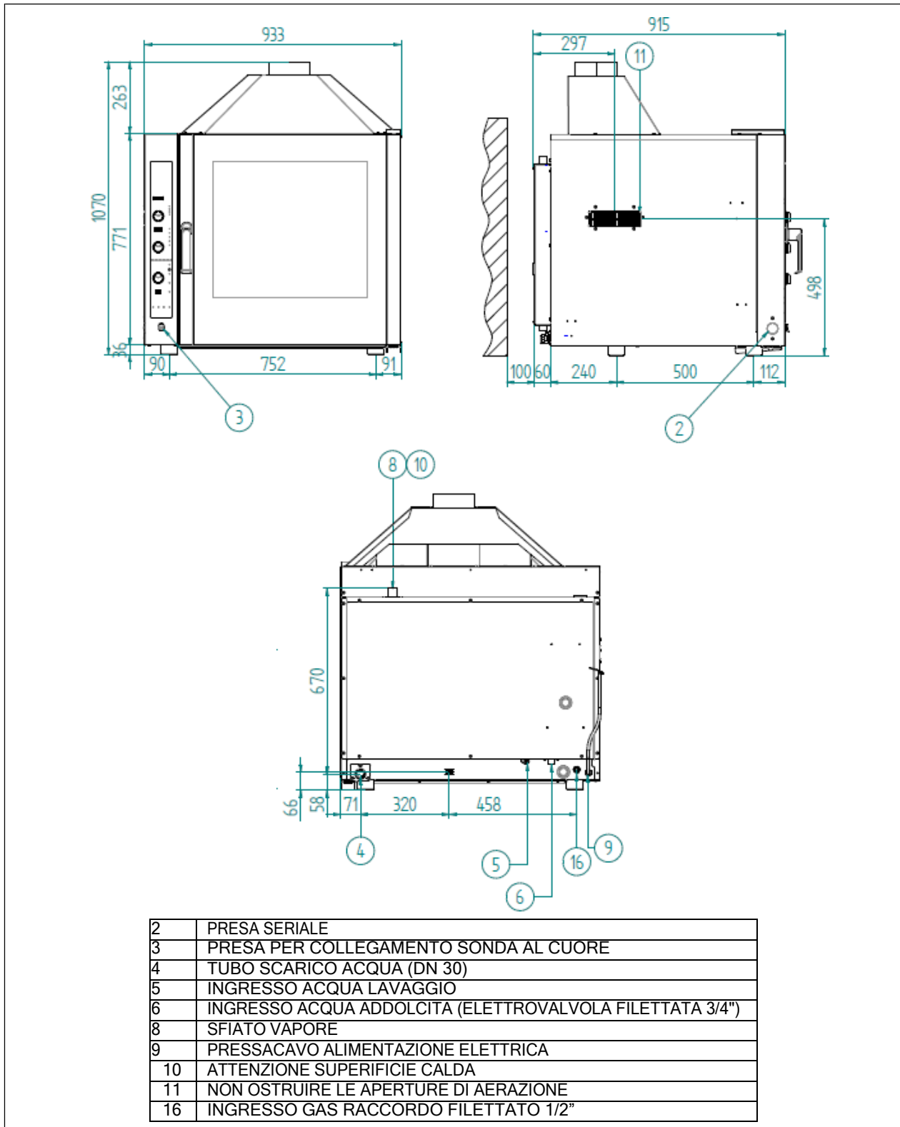
Fig. 3 (Le dimensioni si intendono espresse in mm.)
